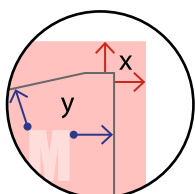
Gestanst eindformaat 37,0 cm x 34,0 cm Toegift van afloop (x) 3 mm Veiligheidsafstand (y) 4 mm
